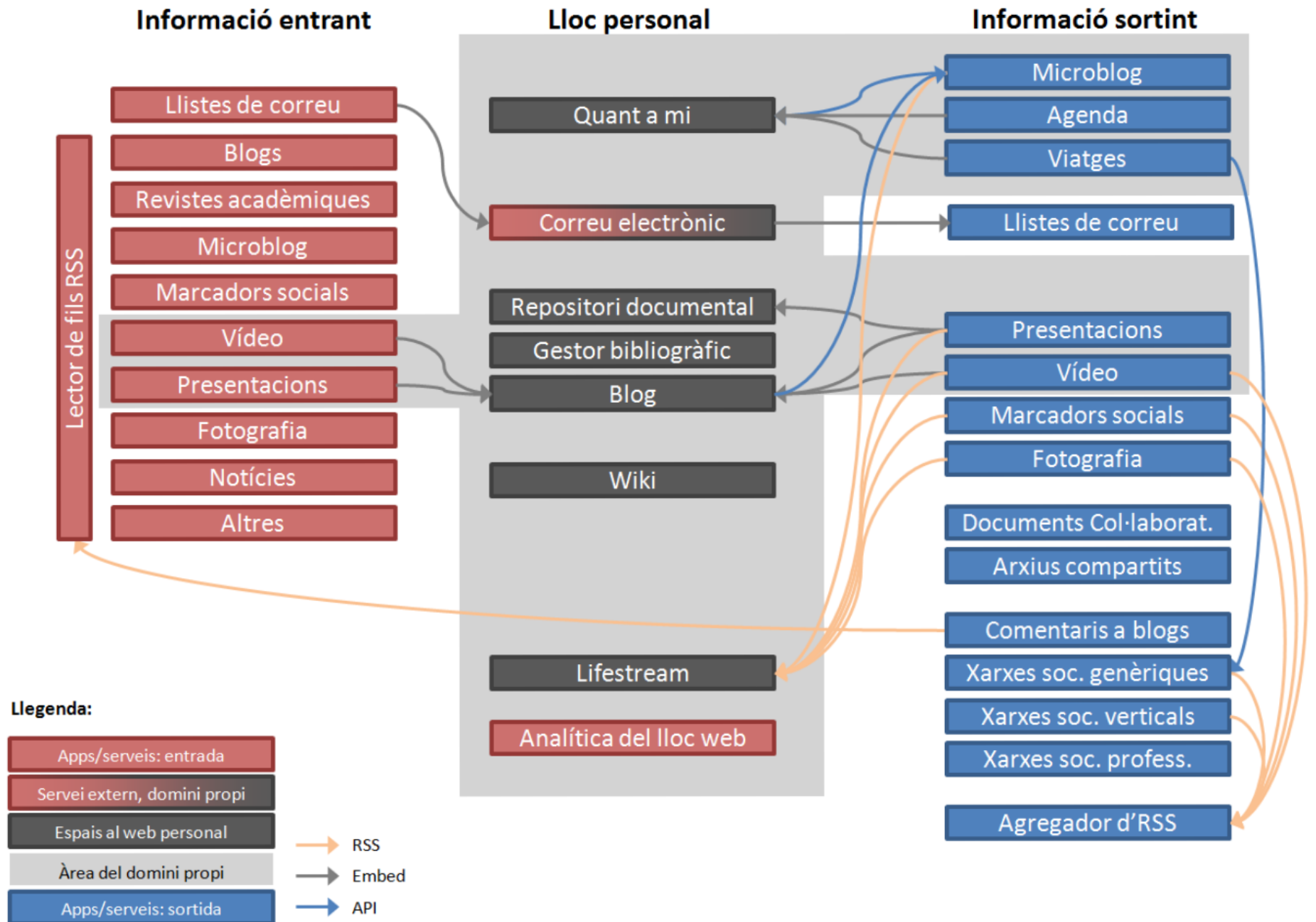
Funcionament d'un Entorn Personal d'Aprenentatge: la infraestructura
